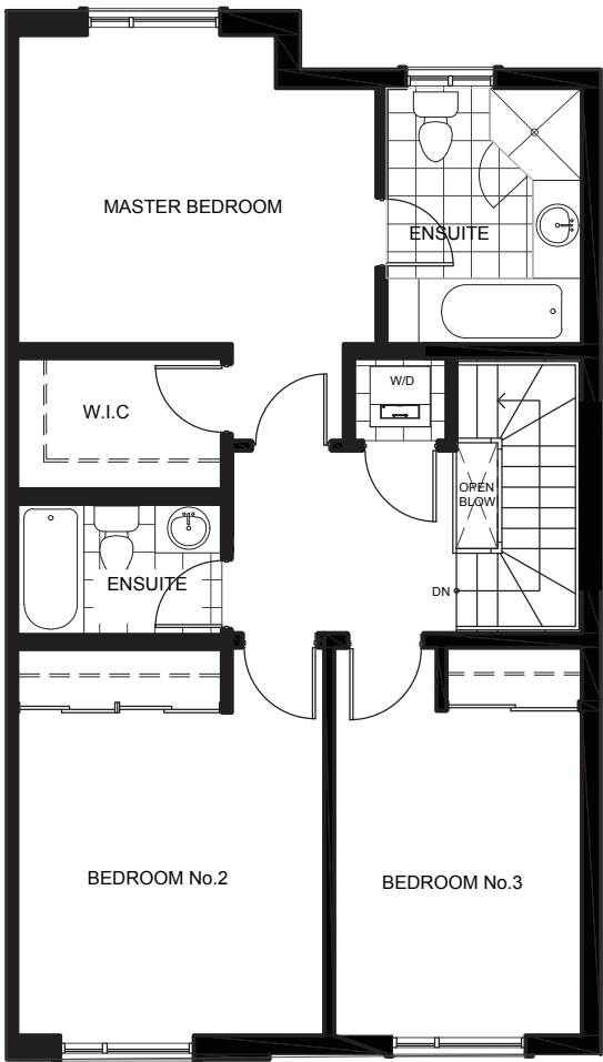
OPTIONAL 3 BEDROOMS
